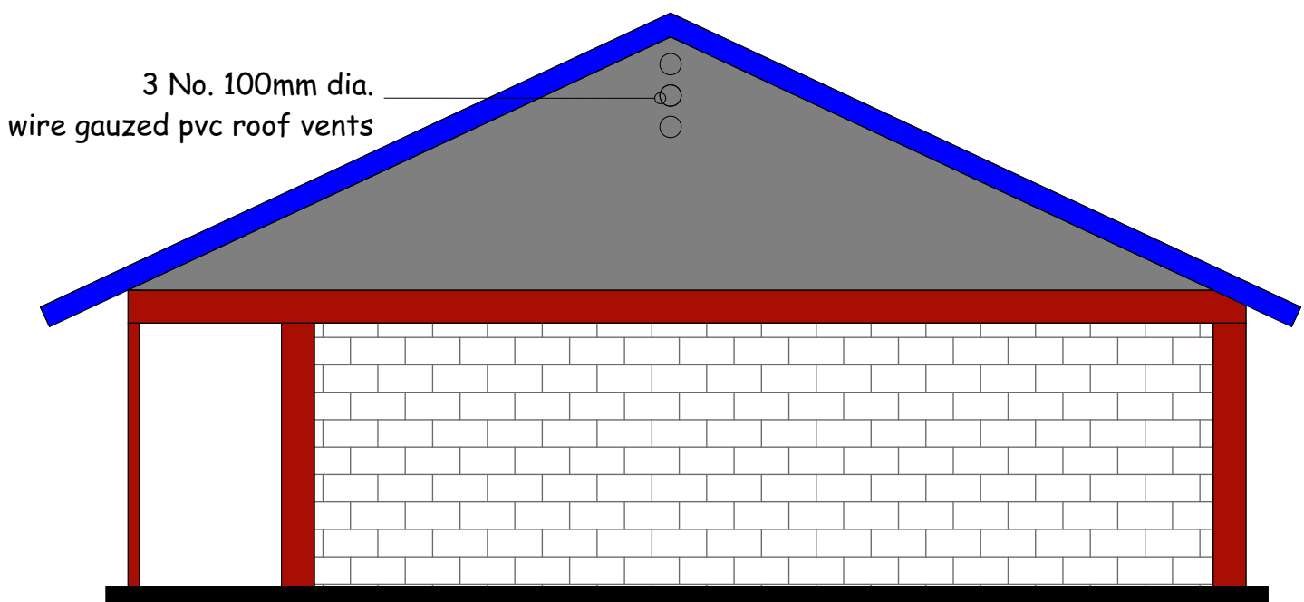
ELEVATION -04-
