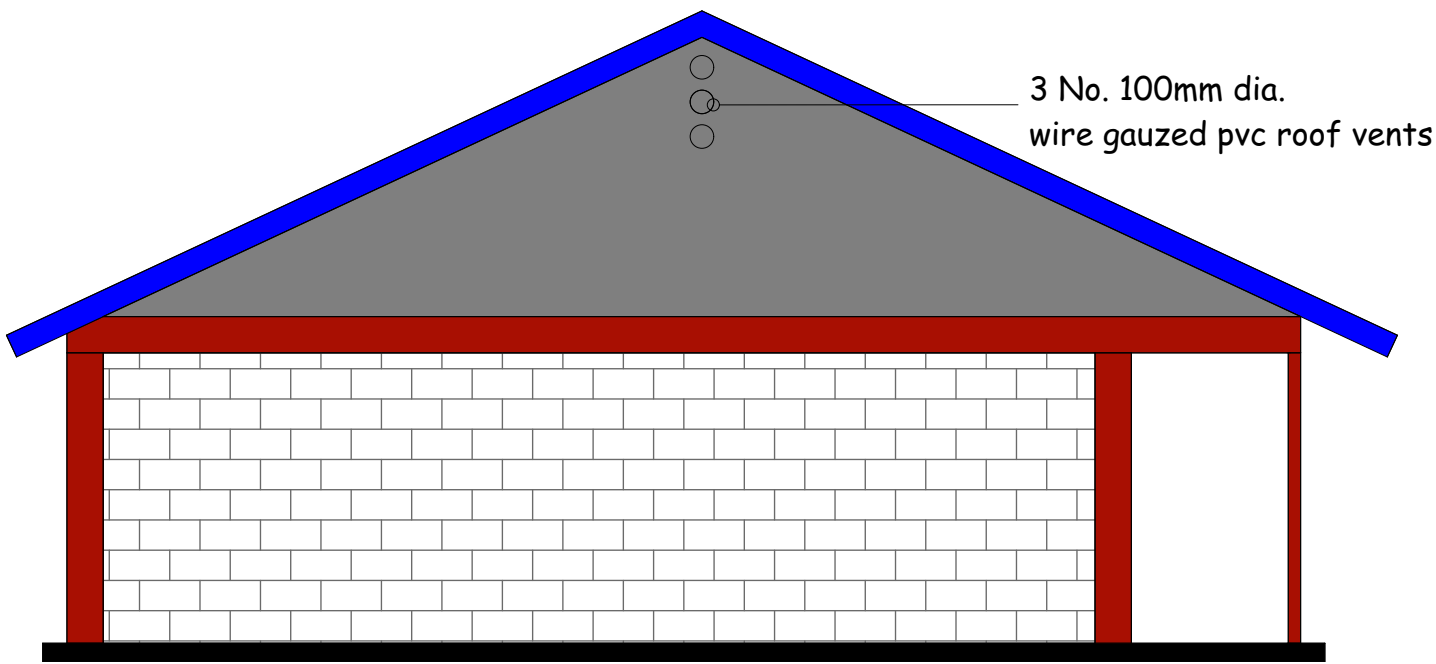
ELEVATION -02-
