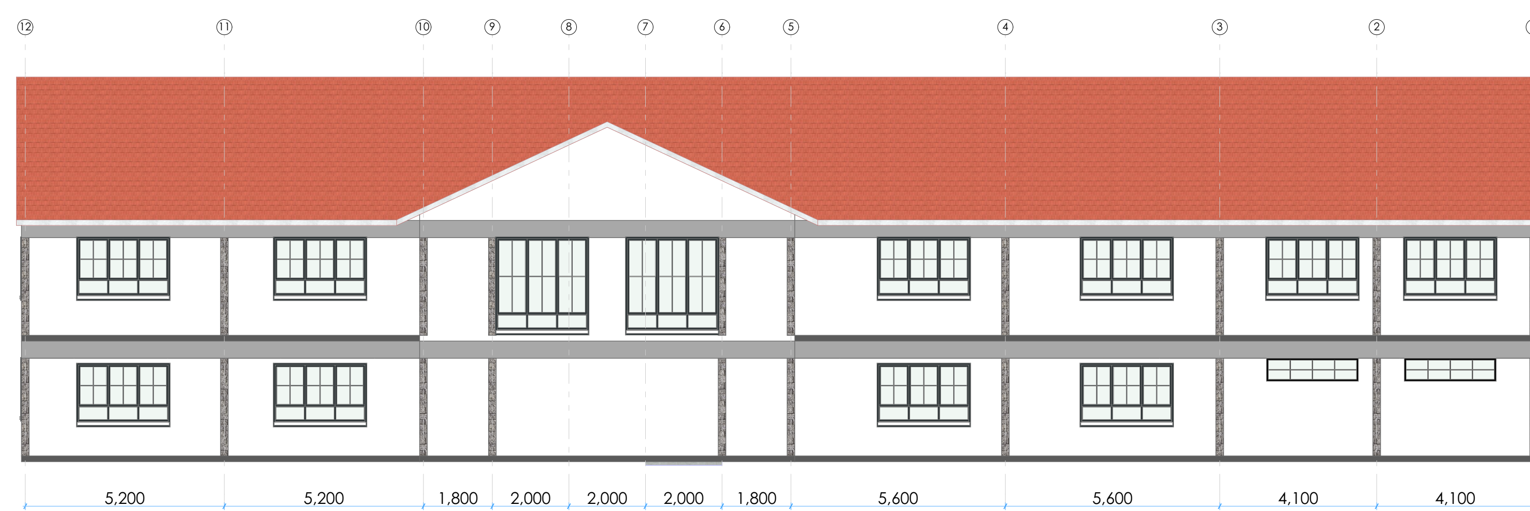
ELEVATION E-3
