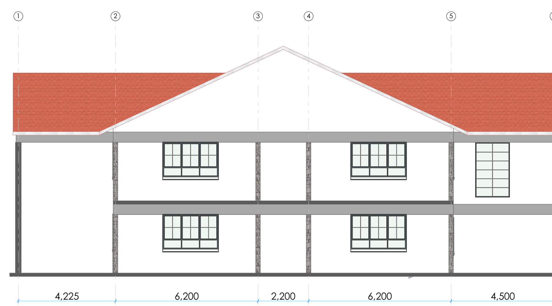
ELEVATION E-4
