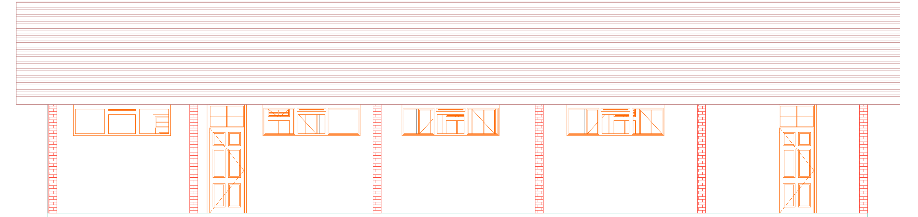
ELEVATION 02
