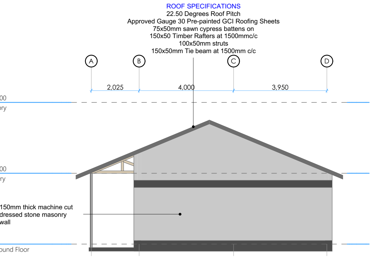
ELEVATION 02 1:100
