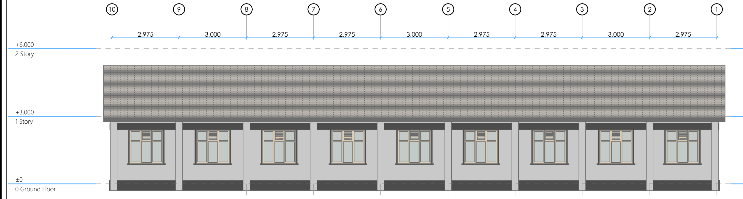
ELEVATION 03 1:100
