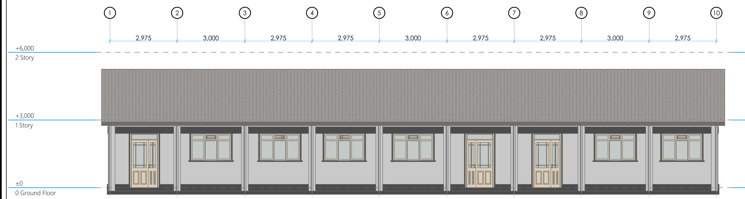
ELEVATION 01 1:100
